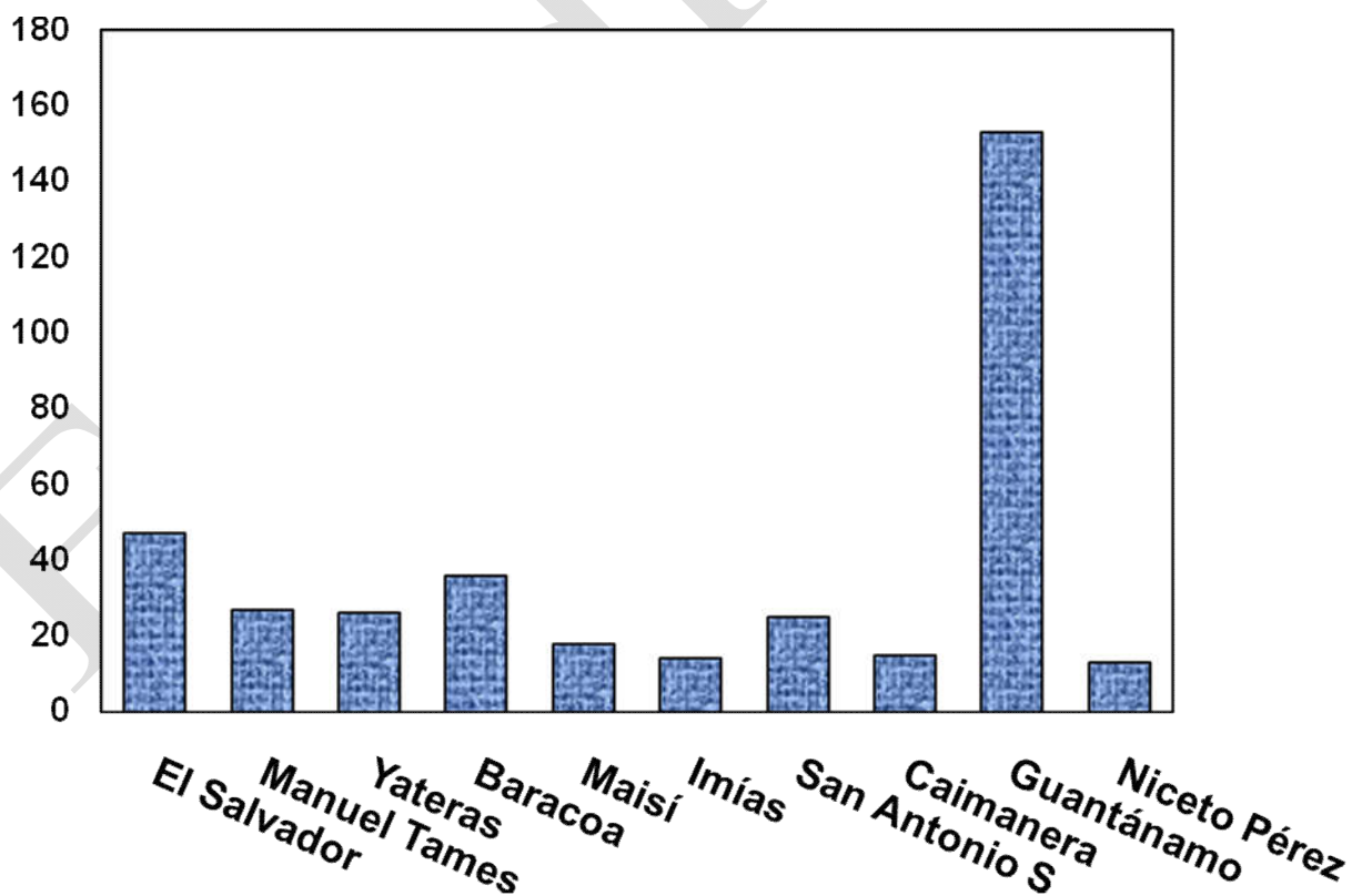
Gráfico 4. Bajo Peso al Nacer según municipios. Provincia Guantánamo. 2016
